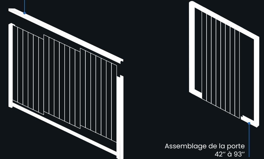
Assemblage du panneau 93 5/16" x 70 1/2" standard
